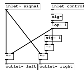
fig 7.7: simple panner
